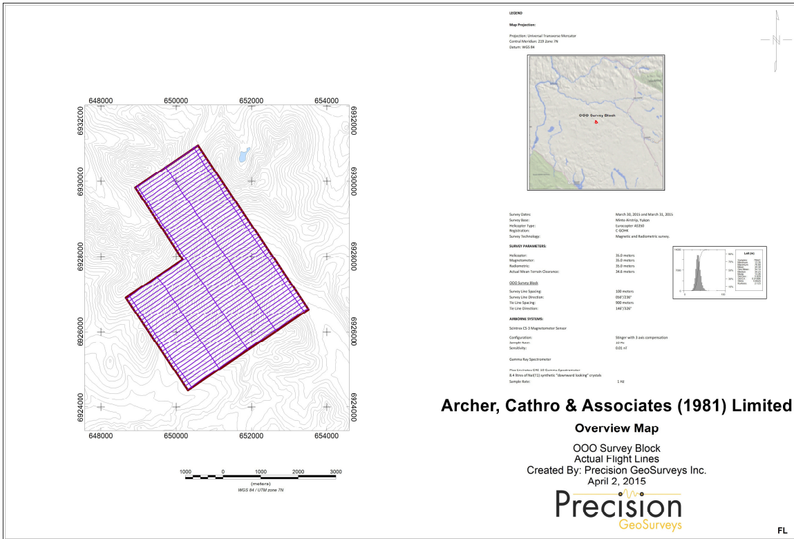
Map 1: OOO survey block actual flight lines.
